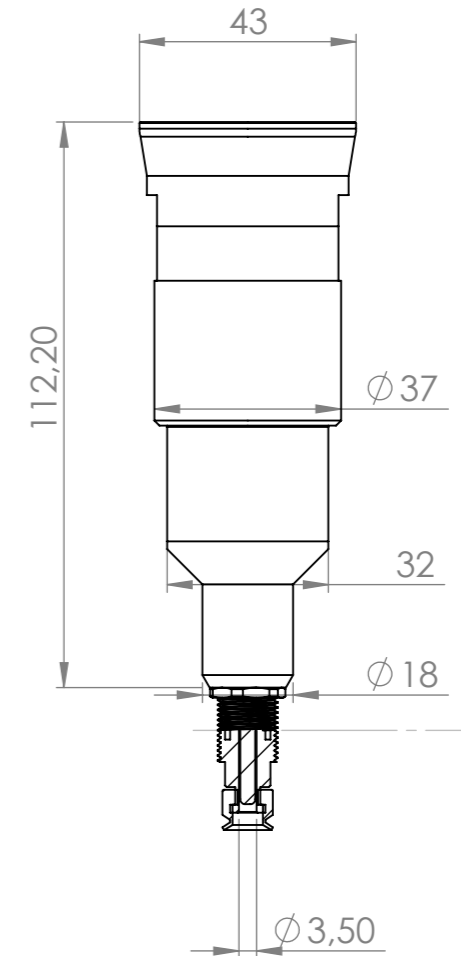
SEZIONE A-A SCALA 1 : 1.5
